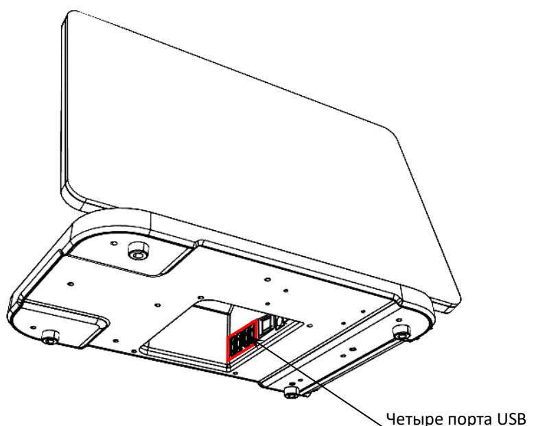
Рисунок 1. Расположение разъемов USB в корпусе смарт-терминала
